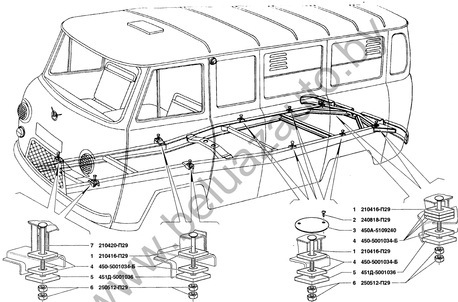
Рис. 145. Подвеска кузова и кабины (5001) Fig. 145. Body and cab mounting (5001)
