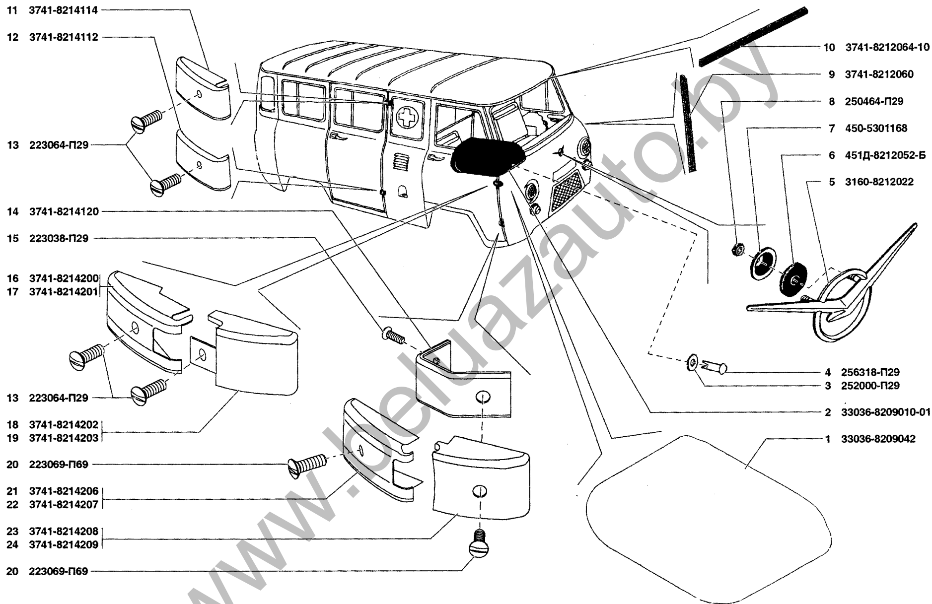
Рис. 176. Чехлы (8209), орнаменты и надписи (8212) Fig. 176. Covers (8209), ornaments and inscriptions (8212)
