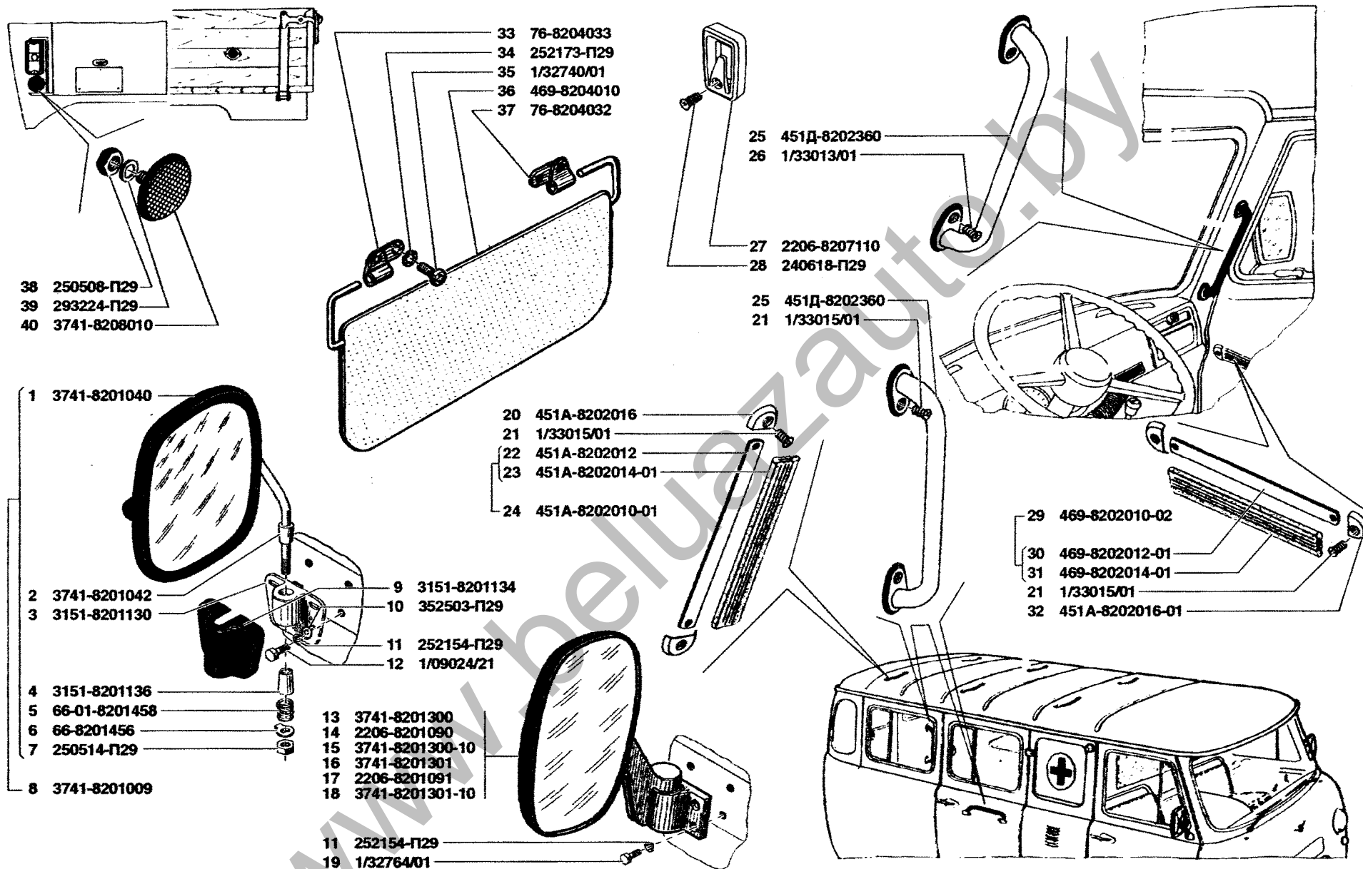
Рис. 175. Зеркало (8201), держатель (поручень) и крючки для одежды (8202), козырек противосолнечный (8204), отражатели света (8208) Fig. 175. Mirror (8201), grab handle and hooks for clothes (8202), sun visor (8204), reflectors (8208)
