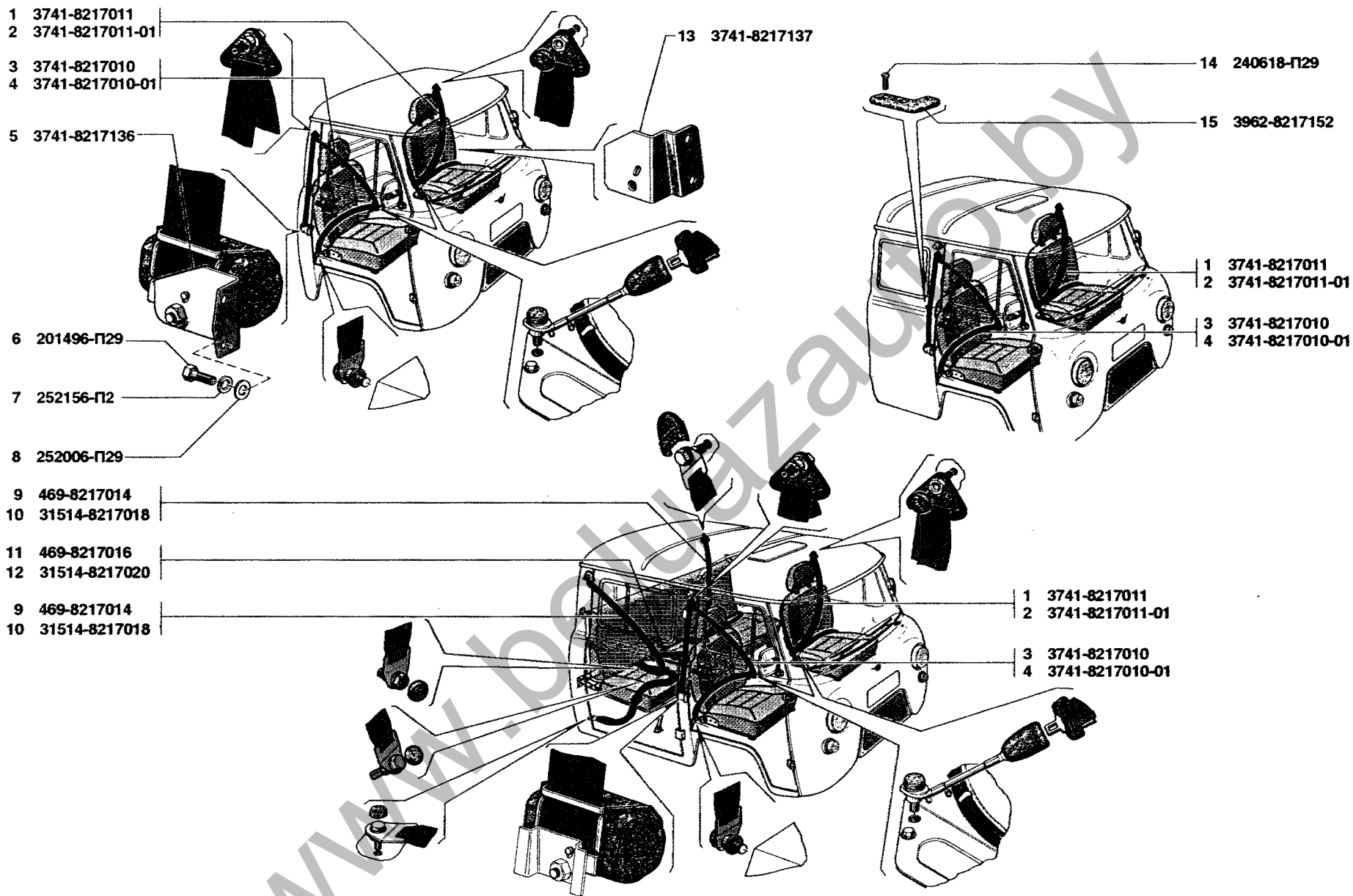
Рис. 177. Ремни безопасности (8217) Fig. 177. Safety belts (8217)
